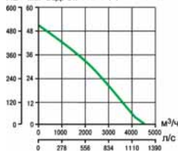
Па мм вод. ст. TRM 50 ED-V 4P
