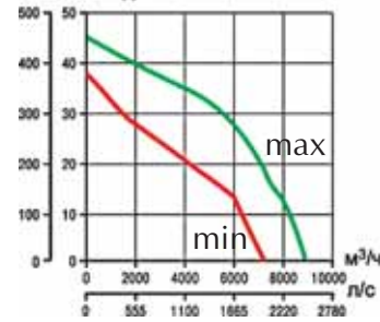
Па мм вод. ст. TRT 100 ED-V 6P
