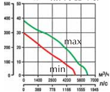
Па мм вод. ст. TRT 70 ED-V 6P
