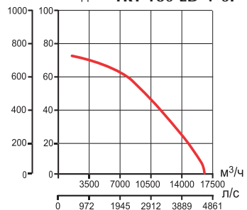
Па мм вод. ст. TRT 180 ED-V 6P
