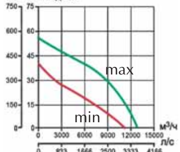
Па мм вод. ст. TRT 150 ED-V 6P
