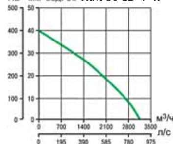
Па мм вод. ст. TRM 30 ED-V 4P
