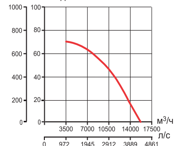
Па мм вод. ст. TRT 210 ED-V 6P
