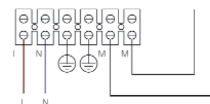
Схема подключения IRM
