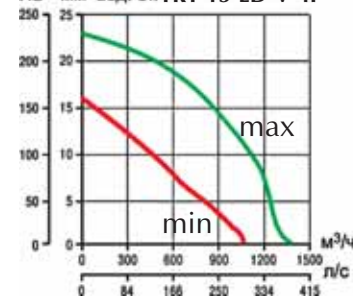
Па мм вод. ст. TRT 15 ED-V 4P
