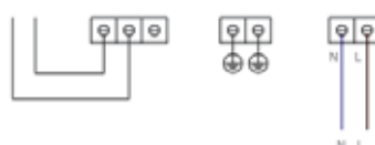
Схема подключения IREM
