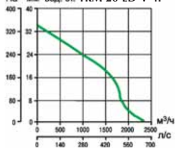
Па мм вод. ст. TRM 20 ED-V 4P
