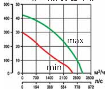
Па мм вод. ст. TRT 30 ED-V 4P
