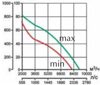
Па мм вод. ст. TRT 100 ED-V 4P
