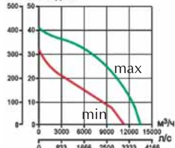
Па мм вод. ст. TRT 150 ED-V 8P
