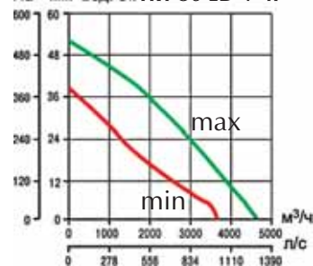
Па мм вод. ст. TRT 50 ED-V 4P
