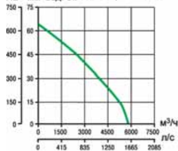
Па мм вод. ст. TRM 70 ED-V 4P
