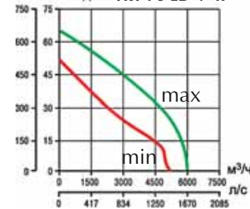
Па мм вод. ст. TRT 70 ED-V 4P
