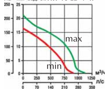
Па мм вод. ст. TRT 10 ED-V 4P
