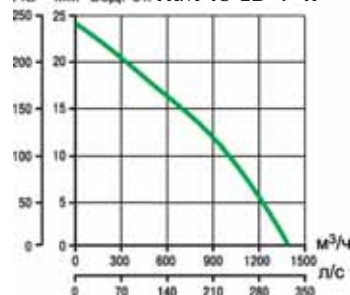
Па мм вод. ст. TRM 15 ED-V 4P
