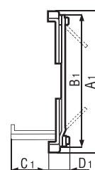
Монтажная рама
