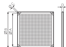
Защитная решетка
