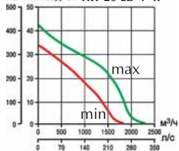
Па мм вод. ст. TRT 20 ED-V 4P
