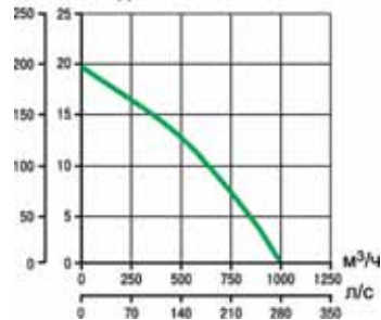
Па мм вод. ст. TRM 10 ED-V 4P
