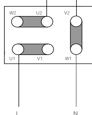
Модели MPM 2 полюса
