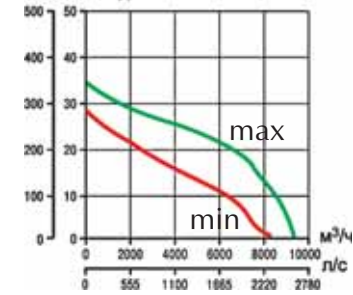
Па мм вод. ст. TRT 100 ED-V 8P
