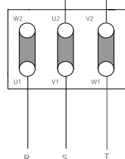
Модели MPM 4 полюса
